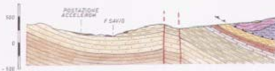
SEZIONE GEOLOGICA A-A' scala 1:50000
