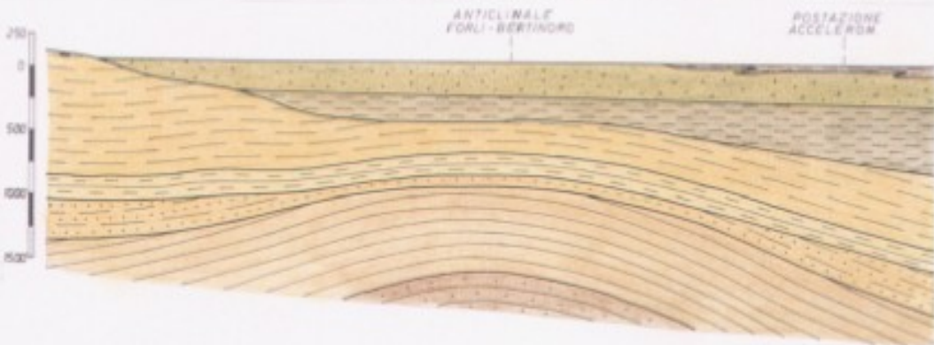
SEZIONE GEOLOGICA A-A' scala 1:50000
