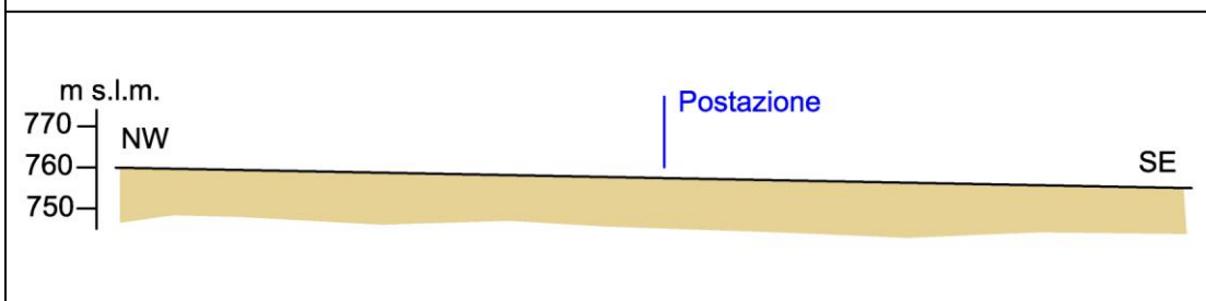
Sezione geologica B-B (scala 1:2.000)
