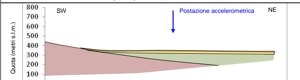
Sezione geologica A-A (scala 1:20.000)
