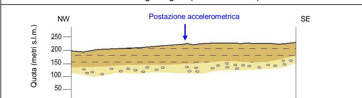
Sezione geologica (scala 1:25.000)
