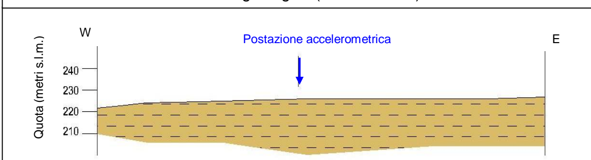
Sezione geologica (scala 1:2.000)
