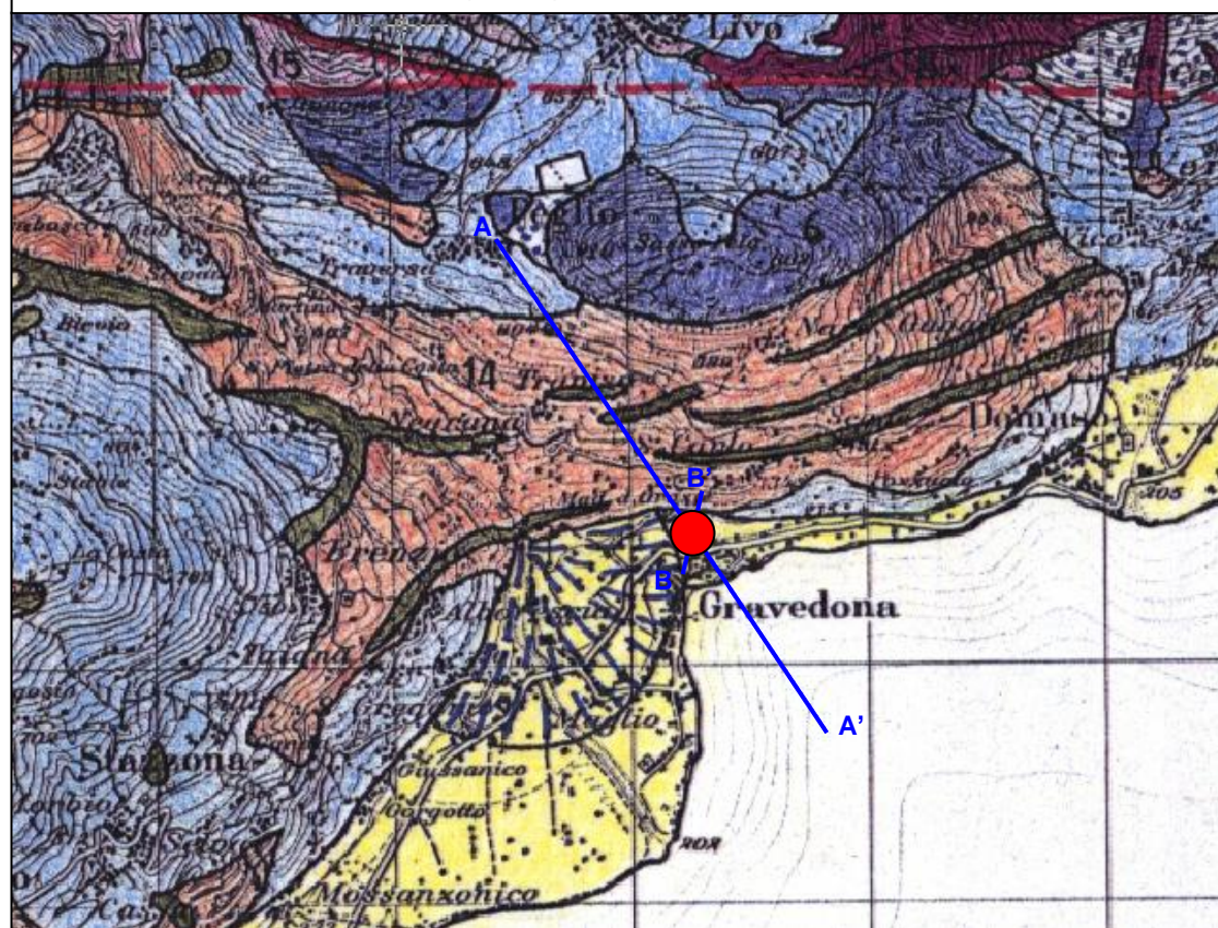
Carta geologica (scala 1:25.000)
