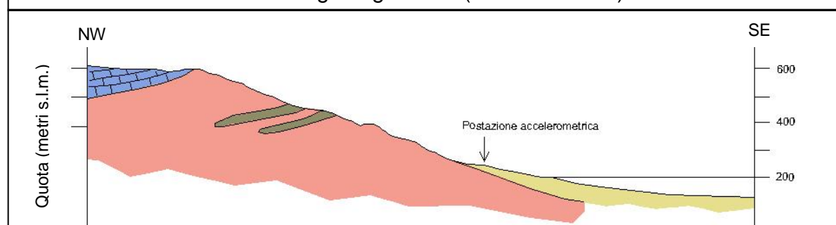
Sezione geologica A-A' (scala 1:20.000)
