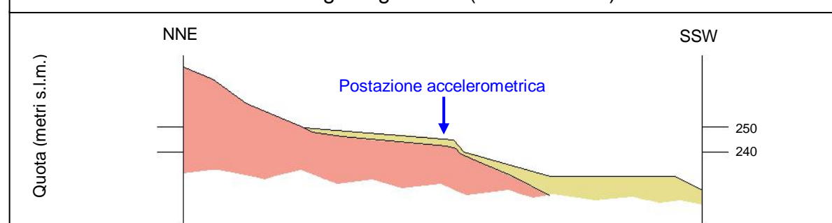
Sezione geologica B-B' (scala 1:2.000)
