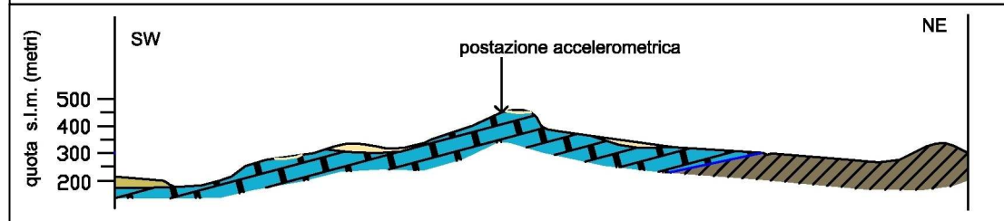
Sezione geologica A – A (scala 1:25.000)
