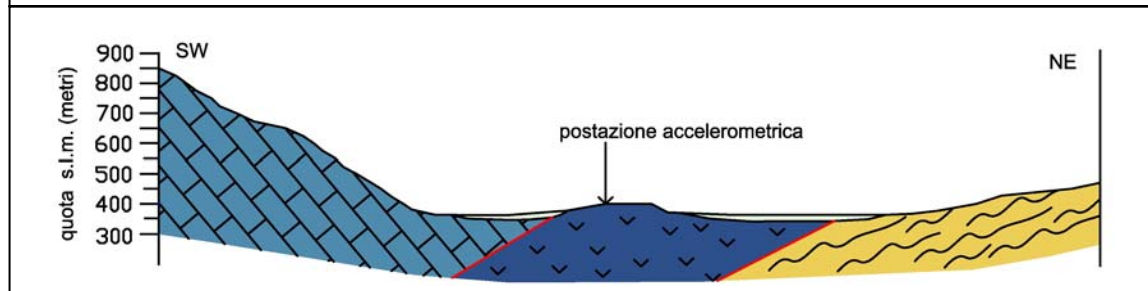
Sezione geologica A-A (scala 1:25.000)
