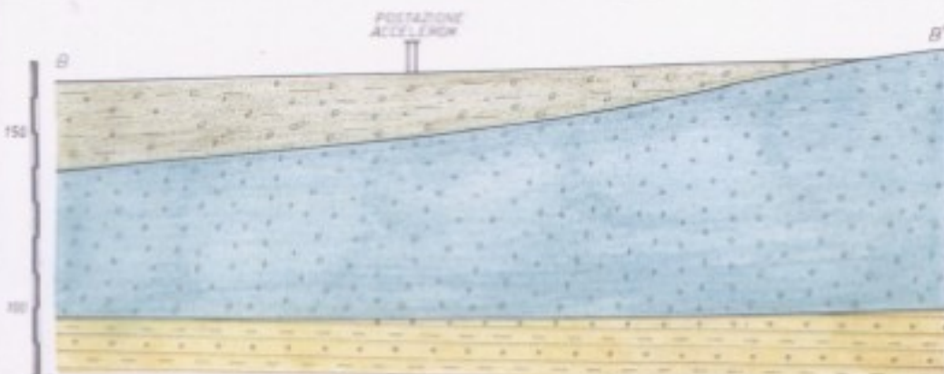
SEZIONE GEOLOGICA B-B' scala 1:2000
