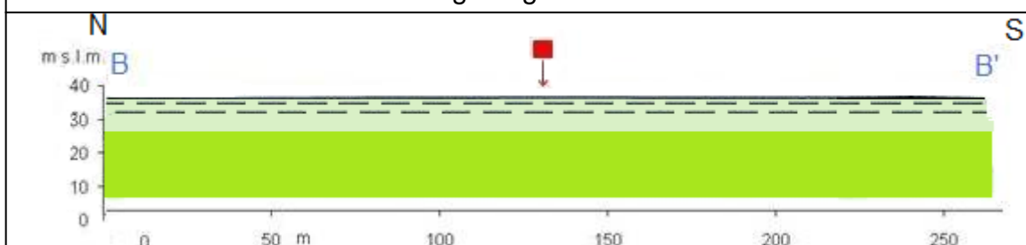
Sezione geologica B-B 1:2.000
