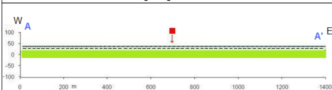
Sezione geologica A-A 1:10.000
